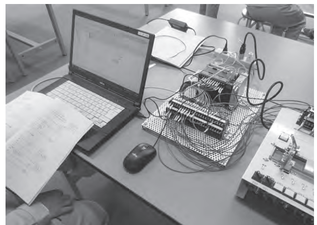
PLC制御実習
